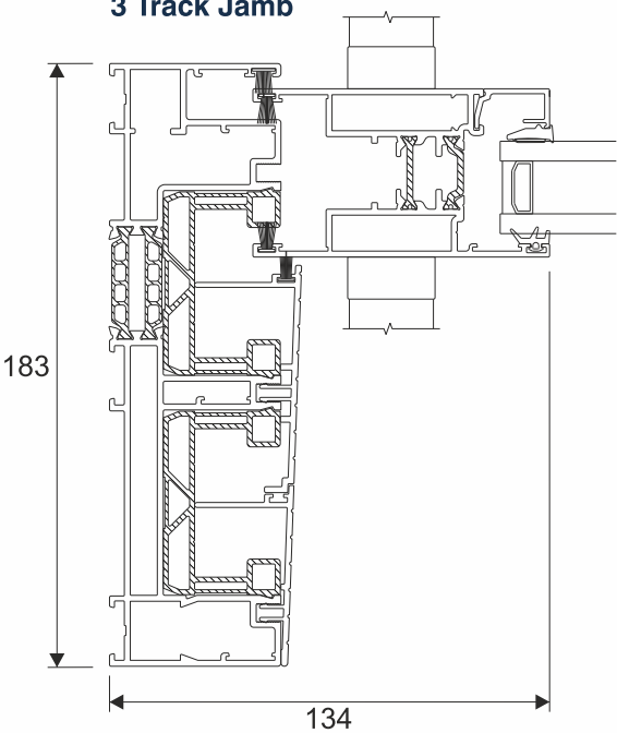
3 Track Jamb
