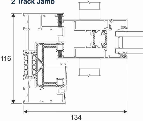
2 Track Jamb
