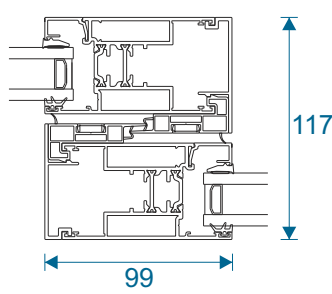
Slim Interlock
