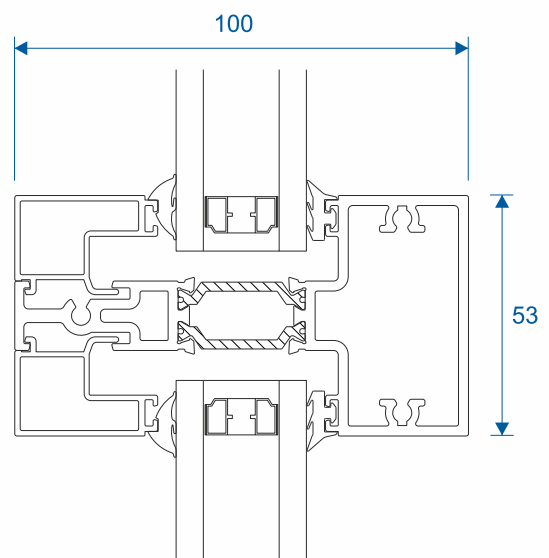
Transom
