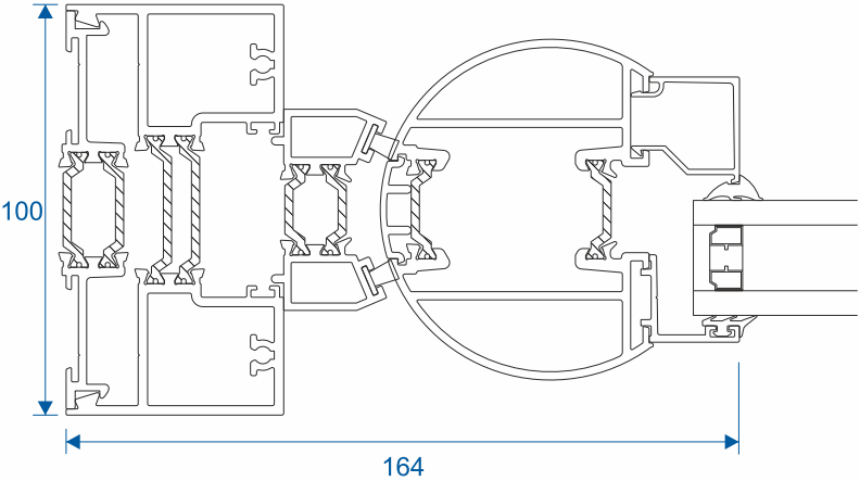
Hinge Jamb
