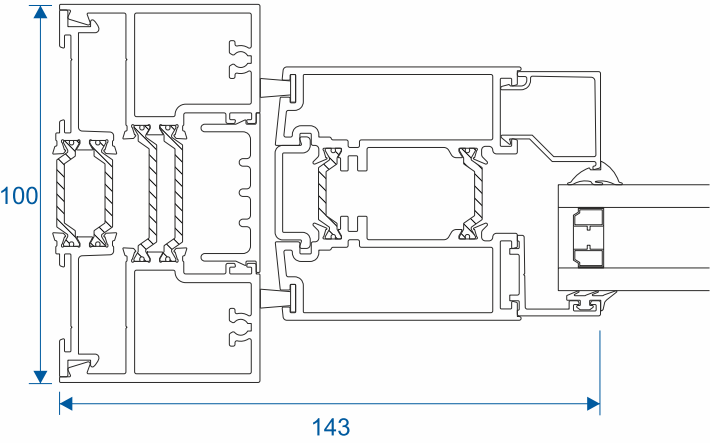
Lock Jamb
